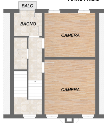
PIANO PRIMO
